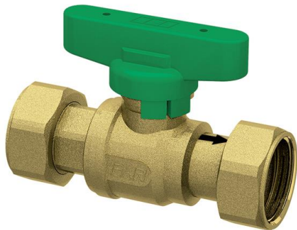
Шаровой кран латунный с накидными гайками и обратным клапаном
