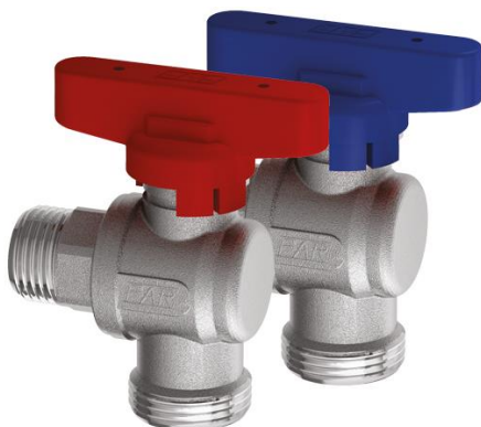
Хромированный угловой запорный шаровой кран - Корпус крана и шар из ковanej латуни CW617N - Хромированный шар - Номинальное давление: 16 бар - Макс. рабочая температура: 95°C - Соединения: Мужское - Мужское соединение: евроконус с плоской вставкой
